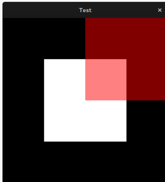
Fig. 4.2: resultado atual
