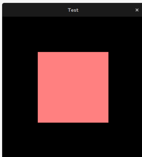
Fig. 4.1: resultado esperado
