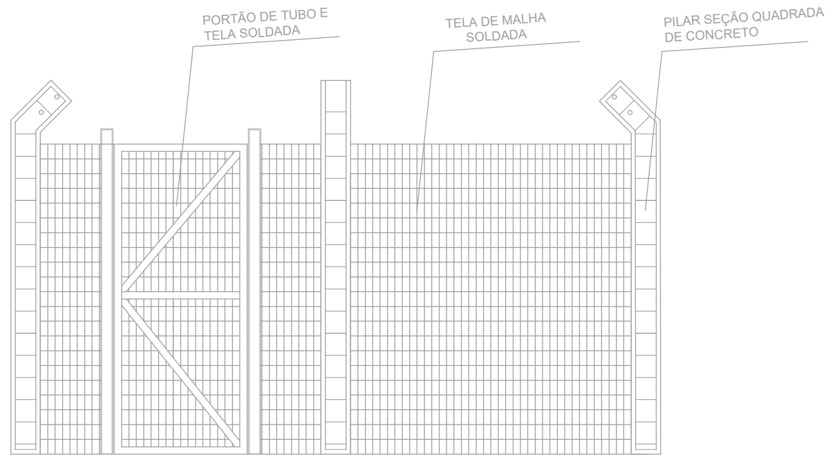
VISTA - FRONTAL
